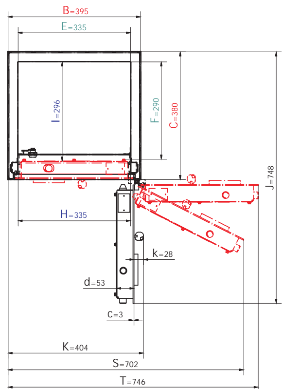
Draufsicht
