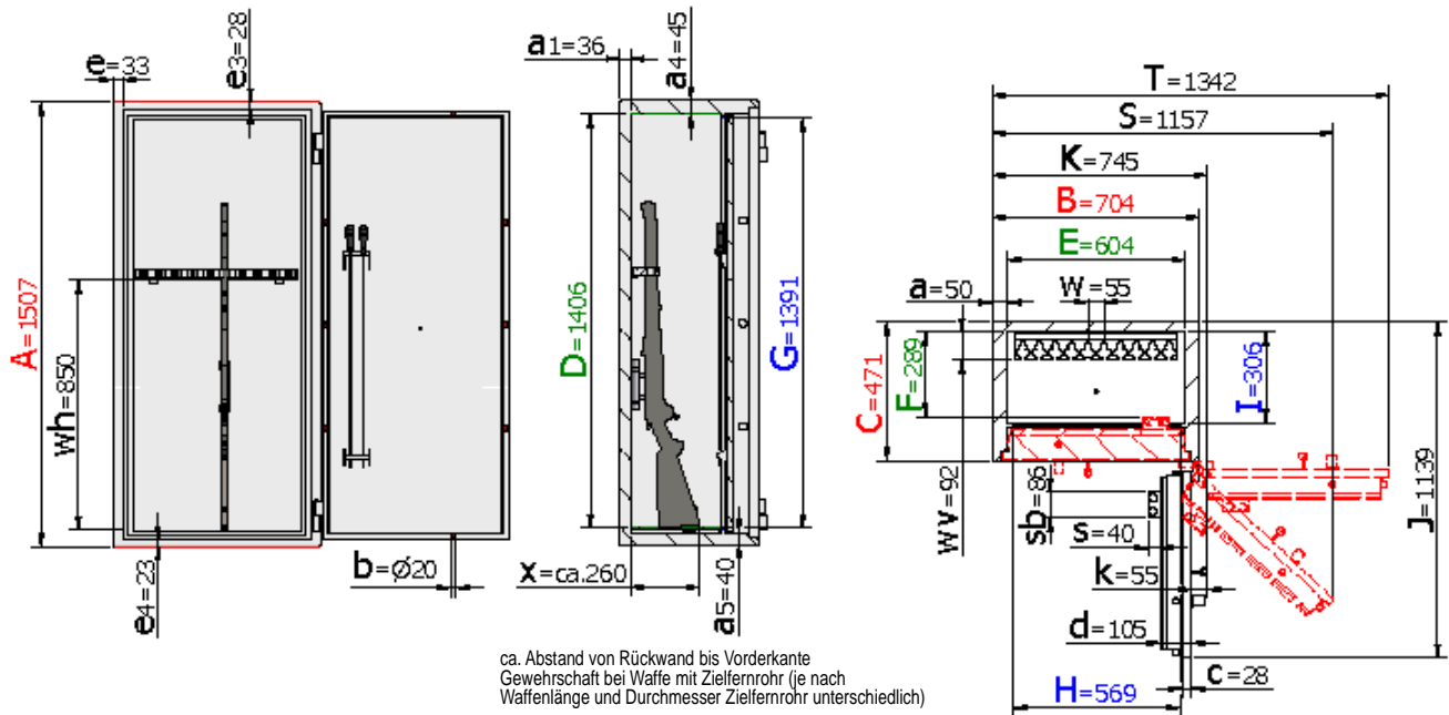
Frontalansicht
